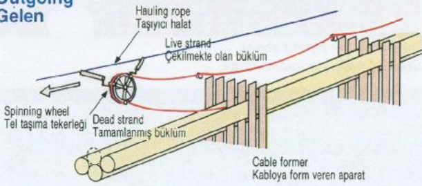
Spinning wheel at the tower top Tel taşıma tekerleği kule tepesinde
