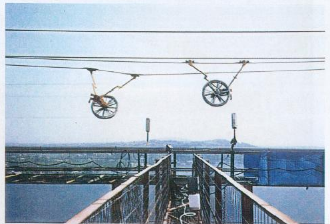
Spinning wheels passing each other at the center of the span Ana açıklığın ortasında buluşan tel taşıma tekerlekleri
