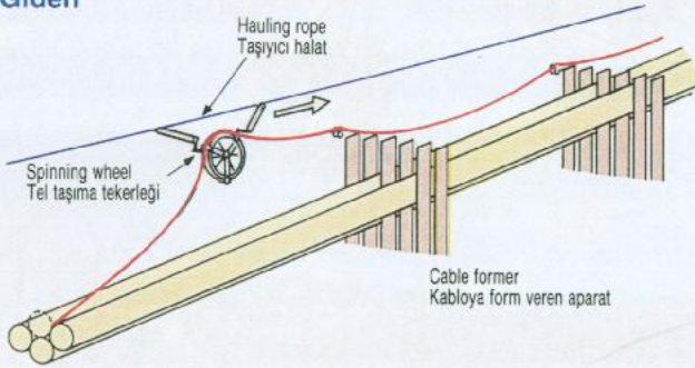
Cable former and preloaded ropes Kablo formunu veren aparat ve ön yük olarak konulmuş halatar
