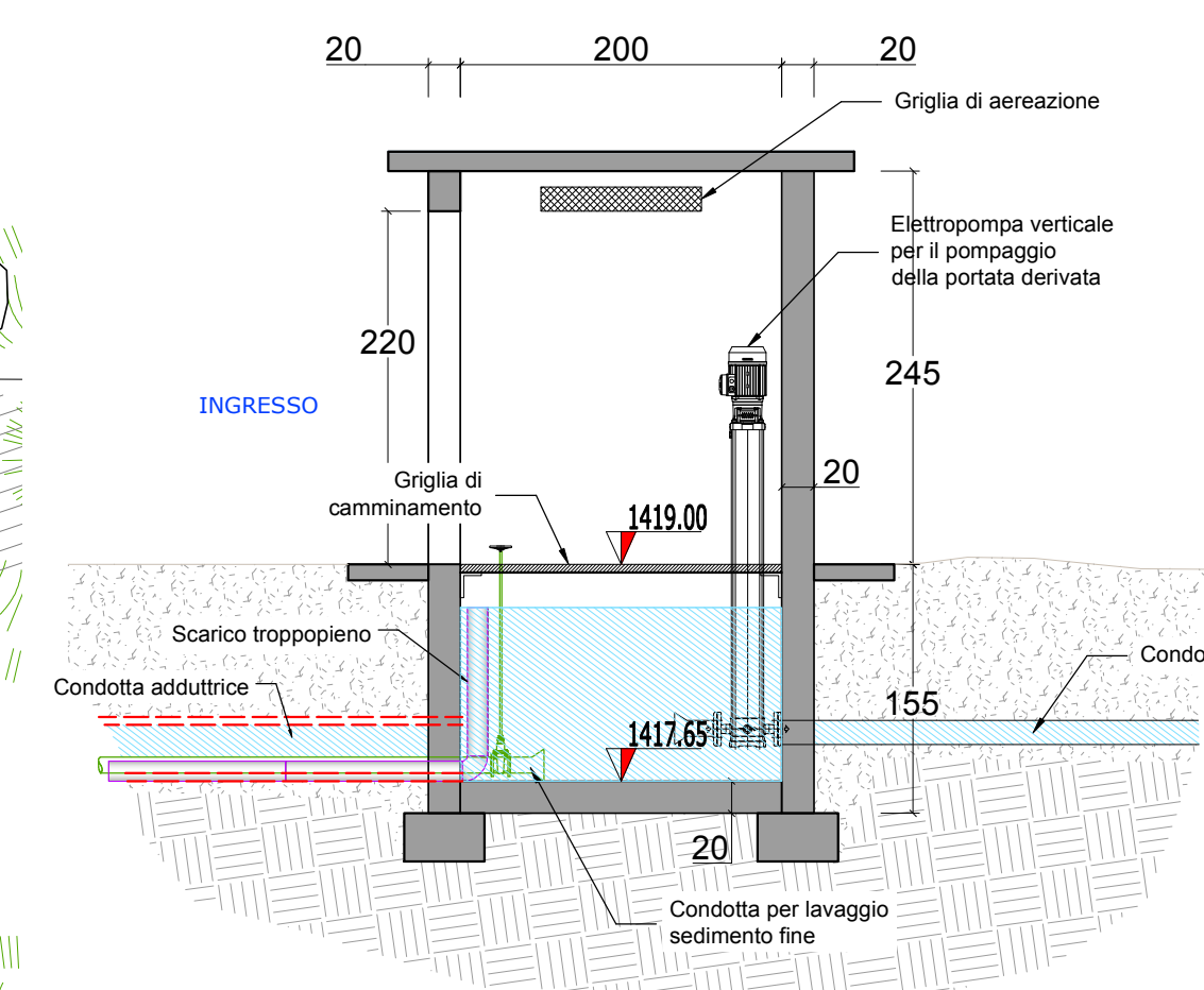
Sezione C-C' (Scala 1:50)
